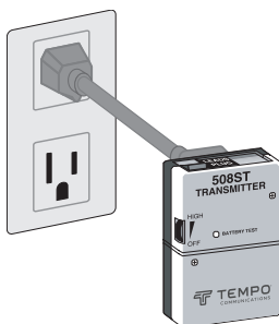
Abb. 01 - Netzadapterstecker
